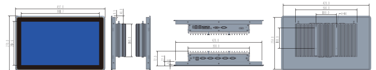
正面 侧面 I/O面 背面
